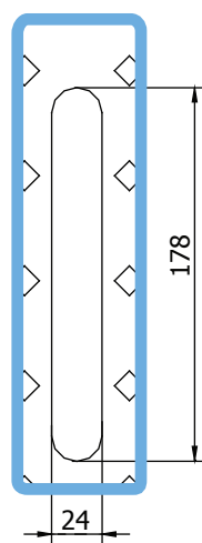
Particolare Fessura
